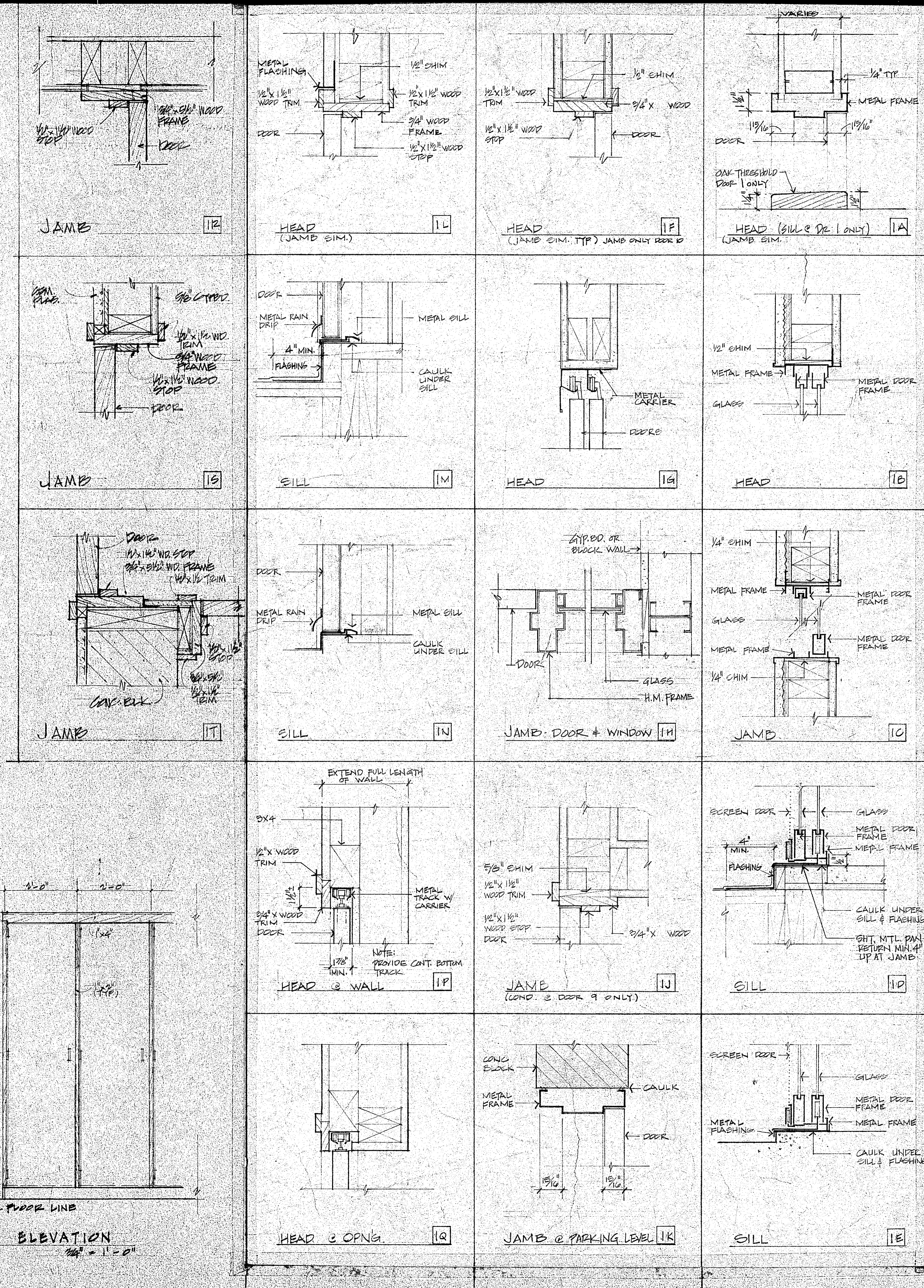
DOOR DETAILS
